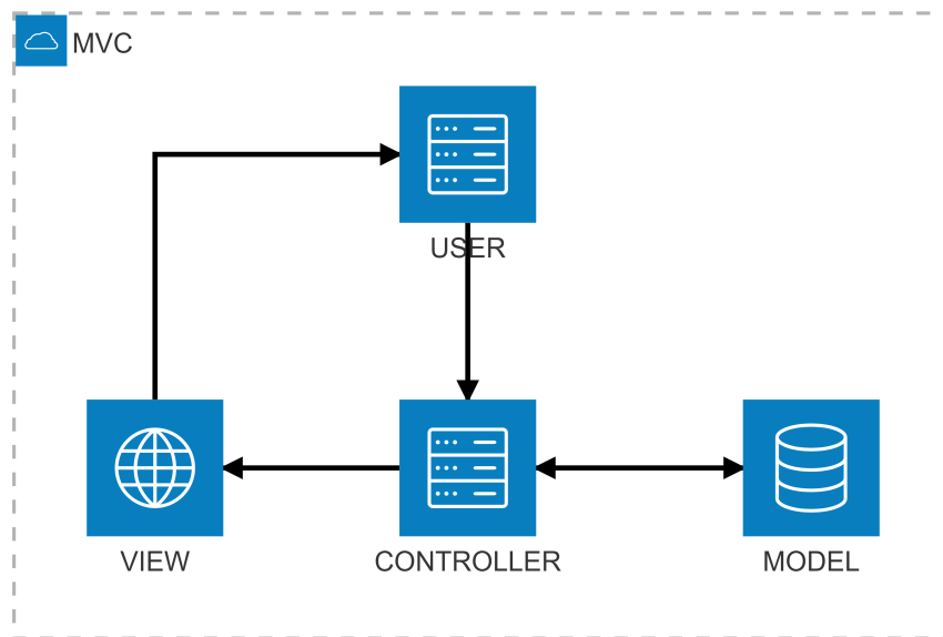
Figura 1 – Arquitetura MVC
